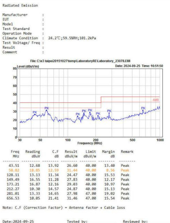
图 4-6 RE 测试垂直方向
